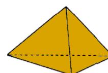
pirâmide de base triangular
