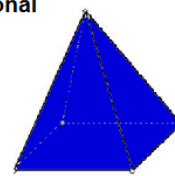
pirâmide de base quadrada
