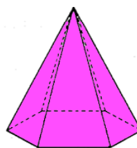
pirâmide de base hexagonal
