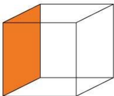
FACE
