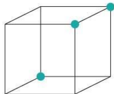
VÉRTICE
